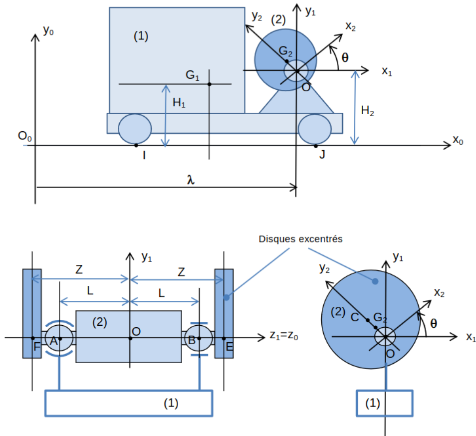
FIGURE 10 – Modélisation de la table vibrante
