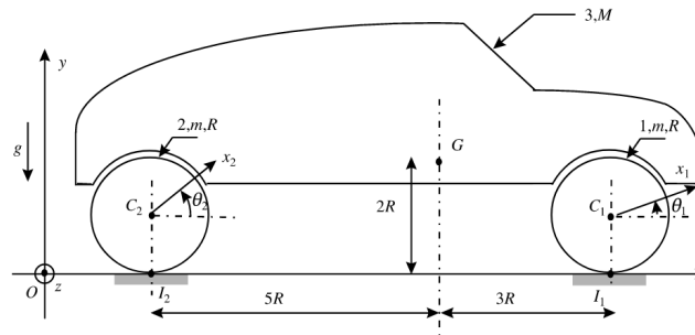
FIGURE 12 – Modélisation du véhicule
