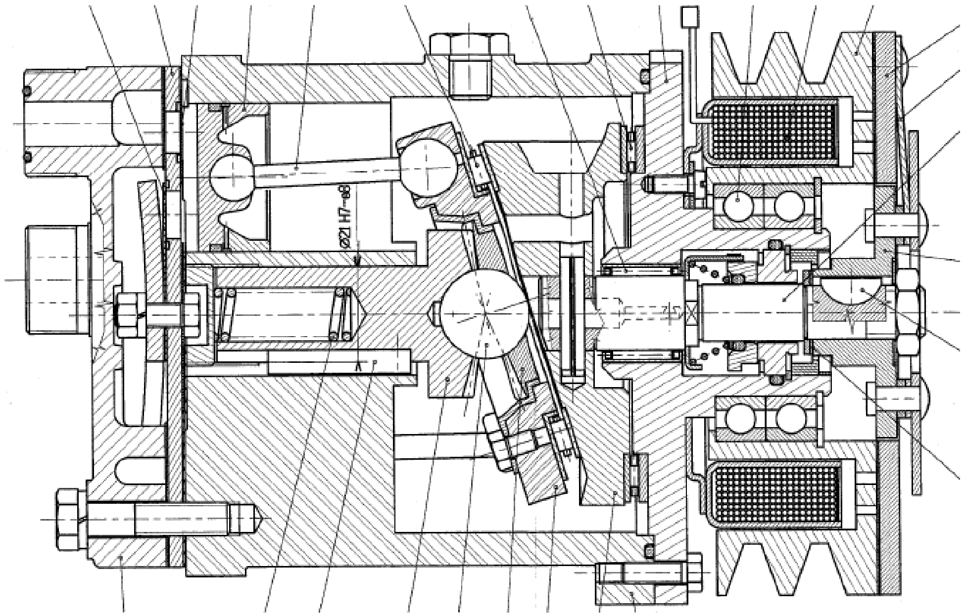
Pompe à 5 pistons axiaux, un seul représenté sur le dessin.
